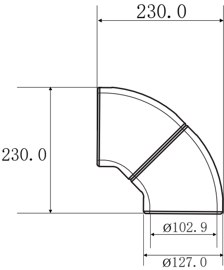
D103 elbow
